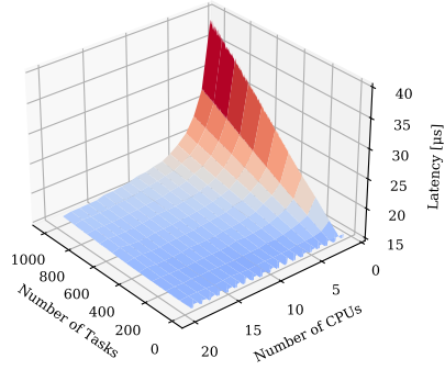
(b) RM Plugin
